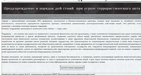
Рисунок 1. Окно ЦОР
