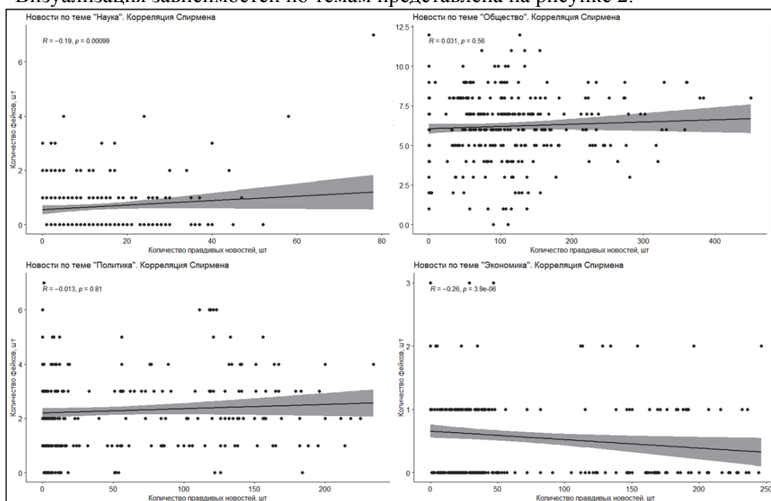
Рисунок 2 - Визуализация зависимостей по темам
